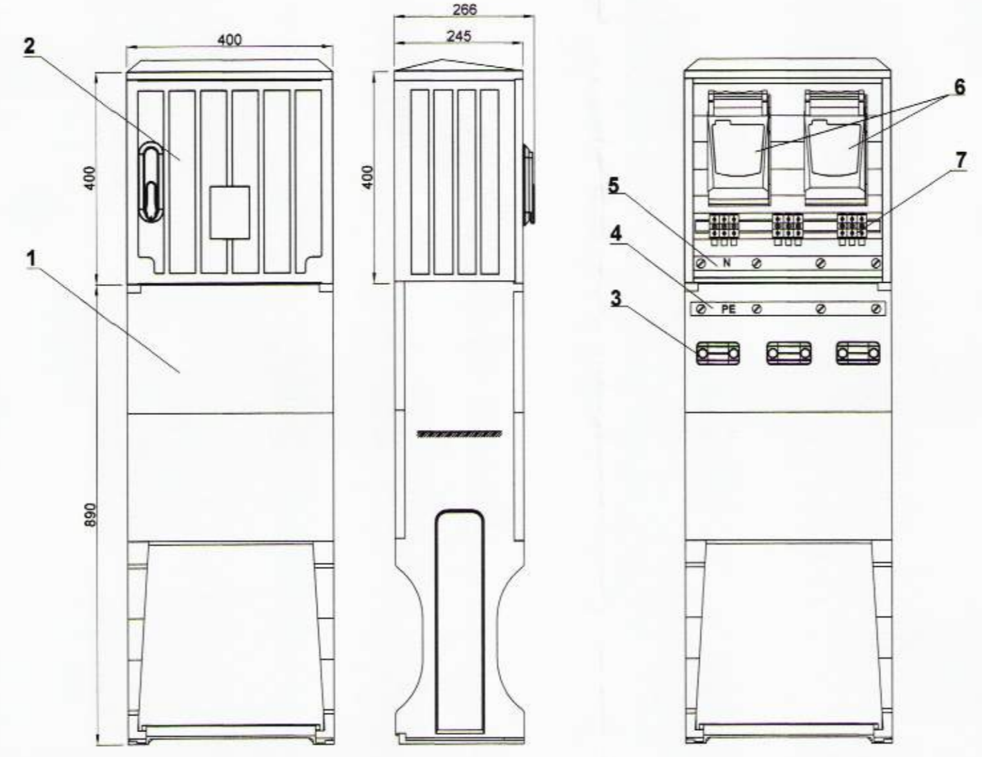
SCHEMAT MONTAŻOWY
