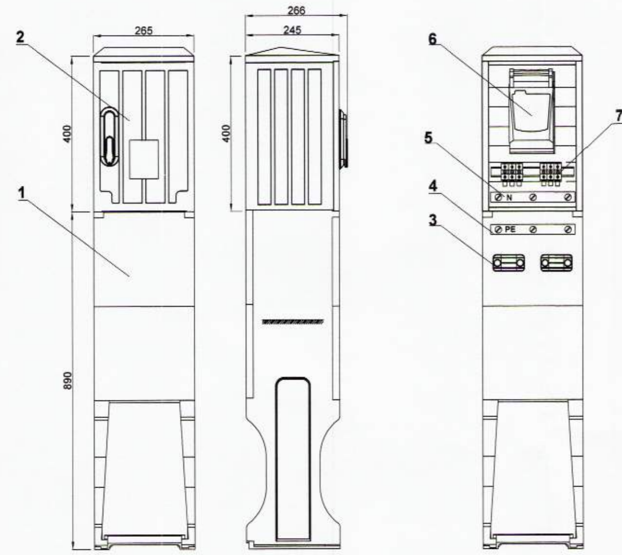
SCHEMAT MONTAŻOWY
