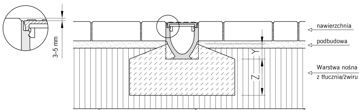
Rys. 2x – schemat wbudowania odwodnienia liniowego w nawierzchnię z bet. kostki brukowej wraz ze szczegółem obniżenia rusztu o ok. 3-5mm poniżej poziomu nawierzchni
