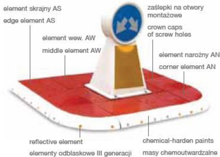
Rys. nr 1 – wyspa z tworzywa sztucznego
