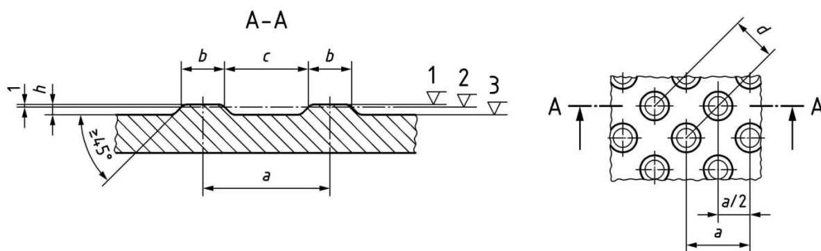
Rys. 2a. Przykładowa płytk ostrzegawcza – szczegół powierzchni
