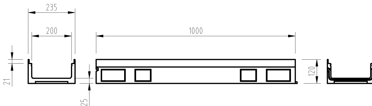
Rys. nr 1x – Przykładowe korytko odwodnienia liniowego szer.23,5cm wys=12cm ( s_k=20\text{cm} oraz h_k=10\text{cm} )
